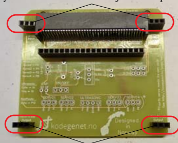
Hylsekontakter for montasje av Neopixler
