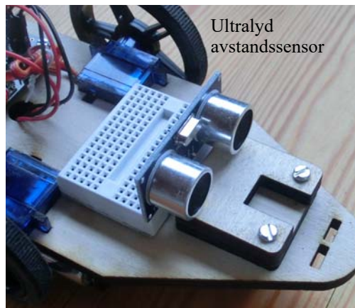
Ultralyd avstandssensor sett bakfra
